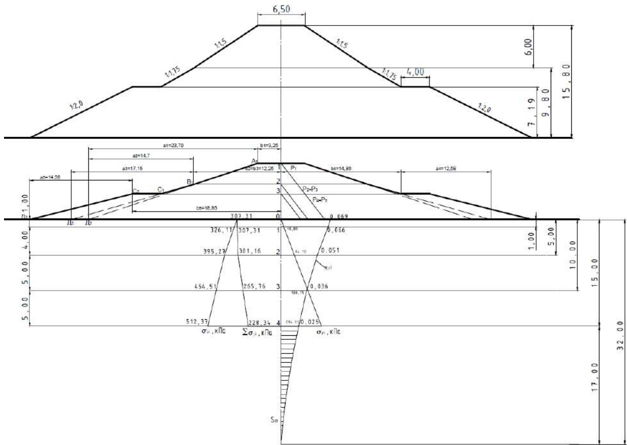
Рис. 1. Расчетная схема для определения напряжений и расчет осадок насыпи.
