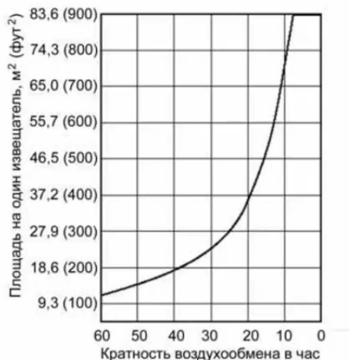
Рис. 2 Зависимость площади защиты точечным дымовым извещателем от кратности воздухообмена в помещении.
