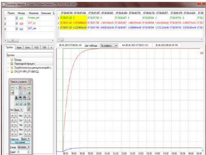
График 5. Временная характеристика при значении K=0.078 с уставкой 160 кгс/см 2
