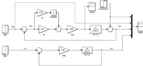
Схема 2. Структурная схема моделирования ОУ с регулятором ПИ ступенчатую функцию с уставкой, 160 кг/см 2
