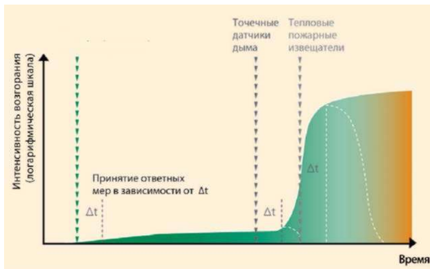
Рис. 1 Сравнение времени обнаружения пожара различными типами пожарных извещателей.
