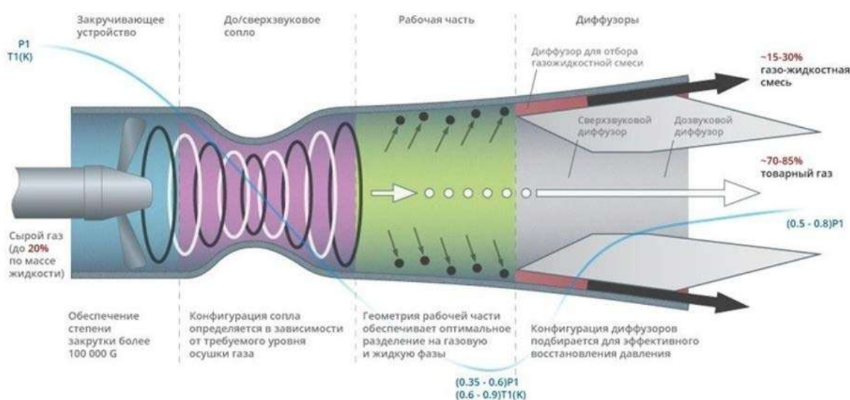
Рис. 1. Принципиальная схема 3S сепаратора.
