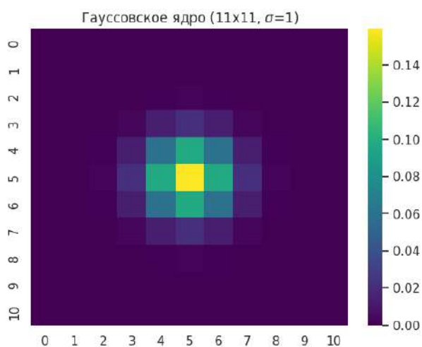
Рис. 5. Визуальное представление гауссова ядра.
