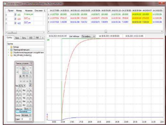
График 6. Временная характеристика при значении K=0.045 с уставкой 180 кгс/см 2
