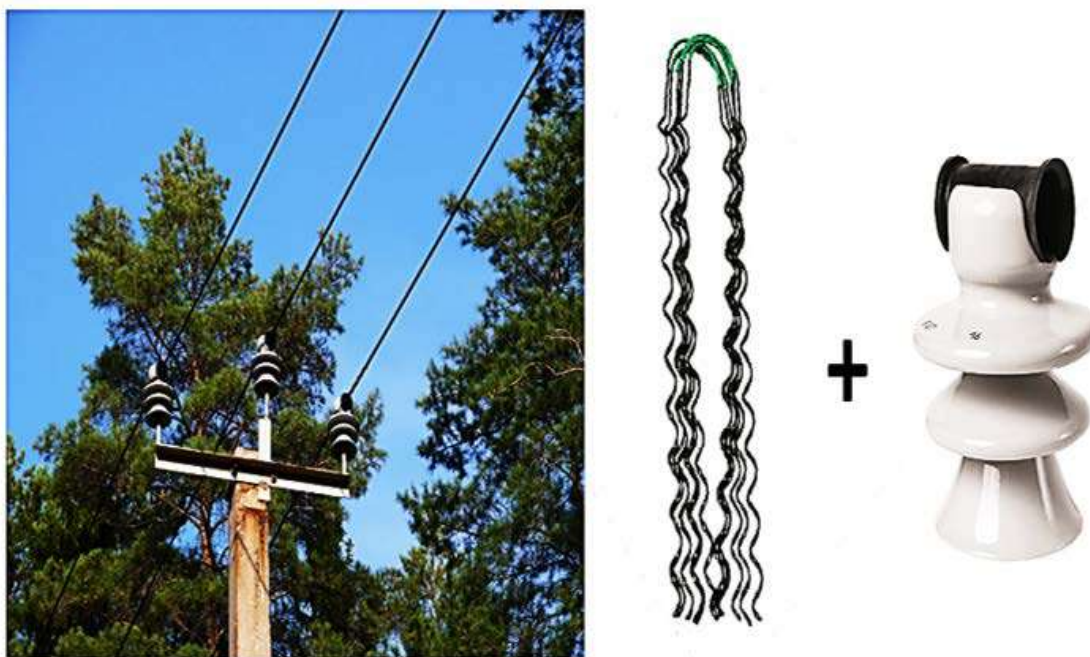
Рис. 1. Существующие конструкции ВЛ 6-20кВ.
