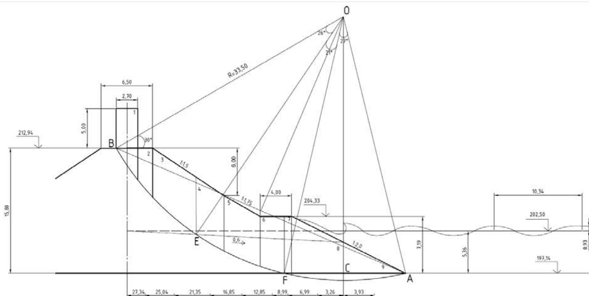
Рис. 1. Расчетная схема для определения устойчивости пойменной насыпи.
