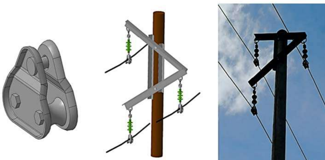
Рис. 2. Конструкция самовосстанавливающейся воздушной линии.
