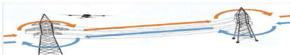
Рис. 1 Схема мониторинга ЛЭП с помощью БАС мультироторного типа.
