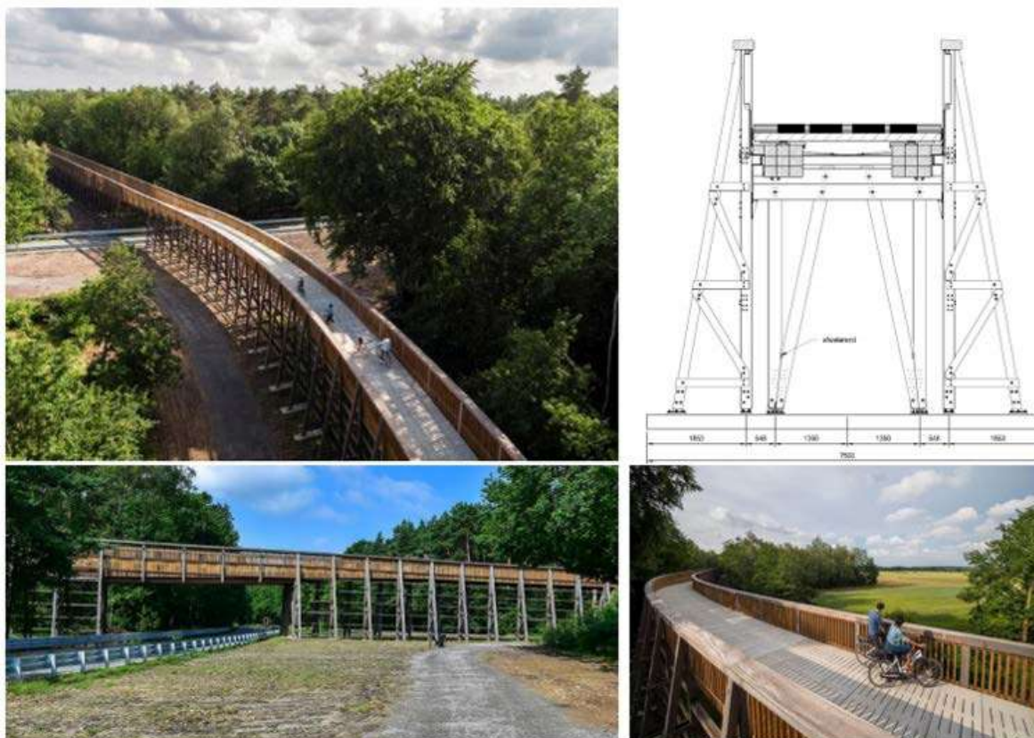
Рисунок 2: Аэрофотоснимок самой высокой секции "Фицен-дор-де-Хайде" вместе с деталями несущих рам главного пролета (вверху), а также вид сбоку на главный пролет и вид с самой высокой точки моста.
