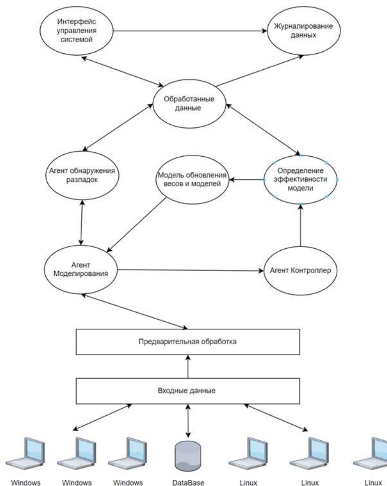
Рисунок 1. Архитектура системы.
