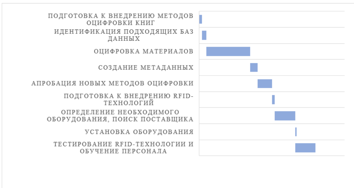
Рисунок 4. Диаграмма Ганта.
