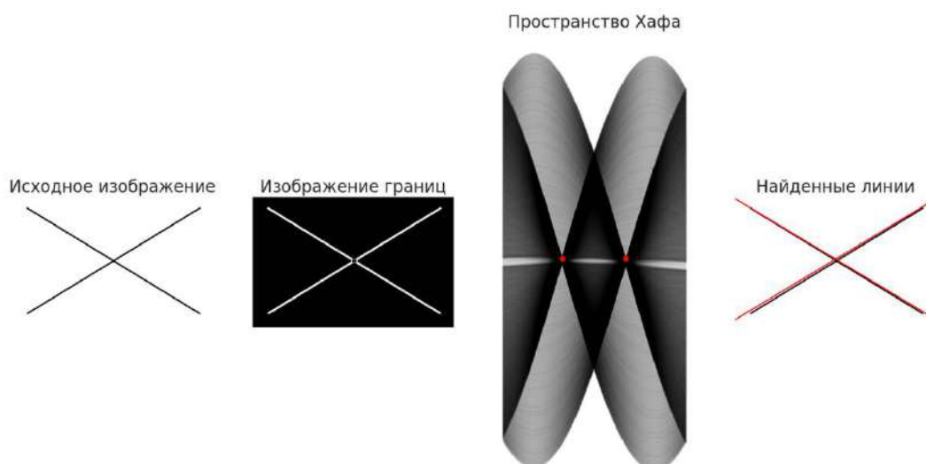
Рис. 11. Принцип работы алгоритма Хафа на примере двух пересекающихся линий.
